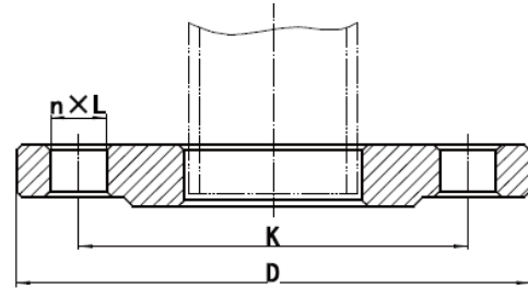
图 6-3 突面（RF）钢制管法兰
