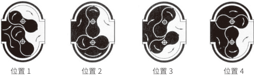
图 1 工作原理图
