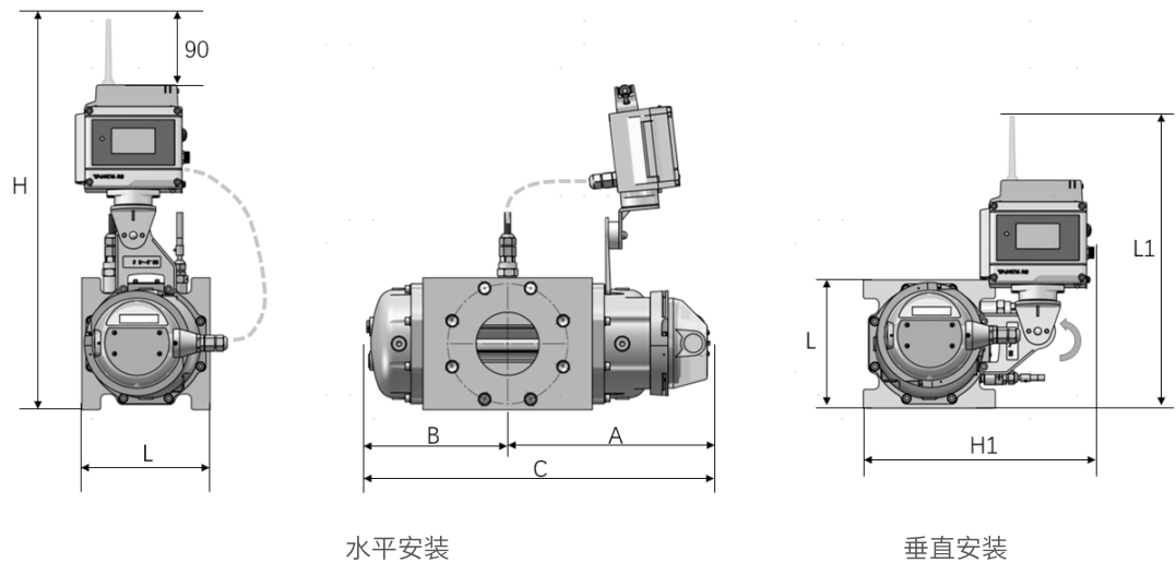
图 5-5 TYL-G □ /TFC-V
