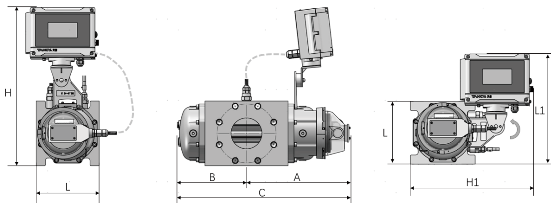
图 5-2 TYL-G □ /FCM
