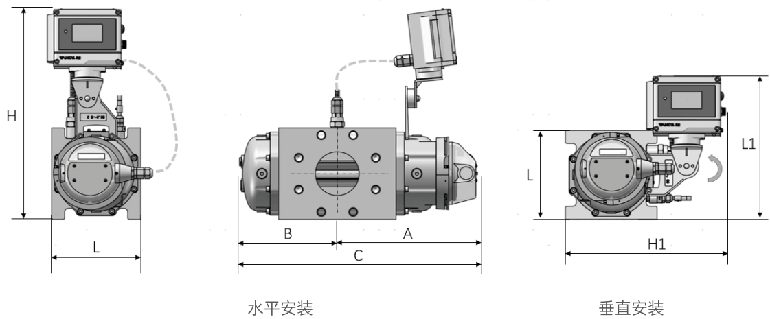
图 5-4 TYL-G □ /FCM-V
