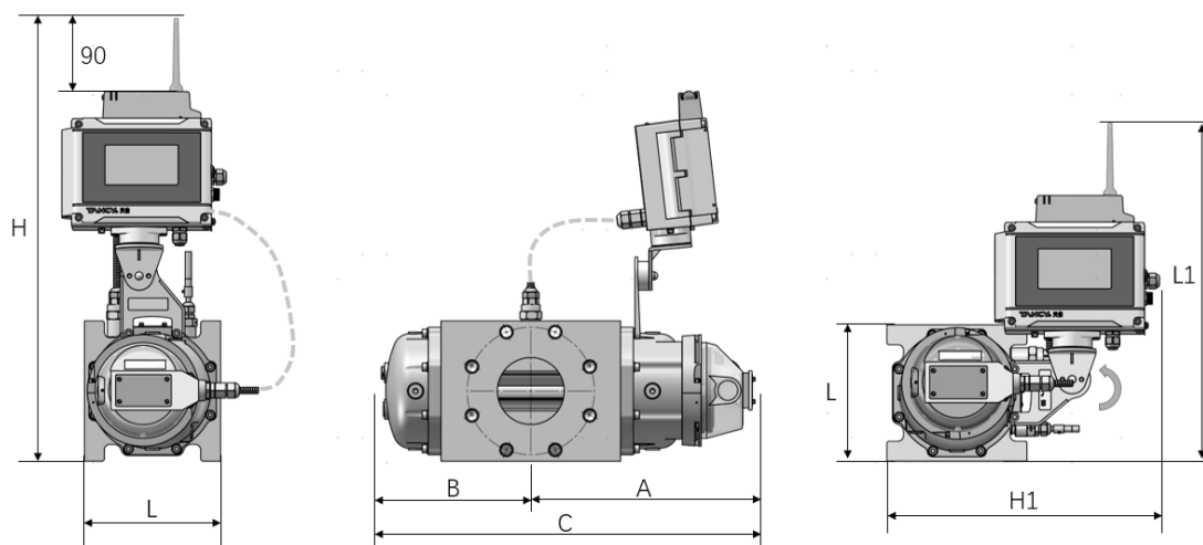
图 5-2 TYL-G □ /FCM
