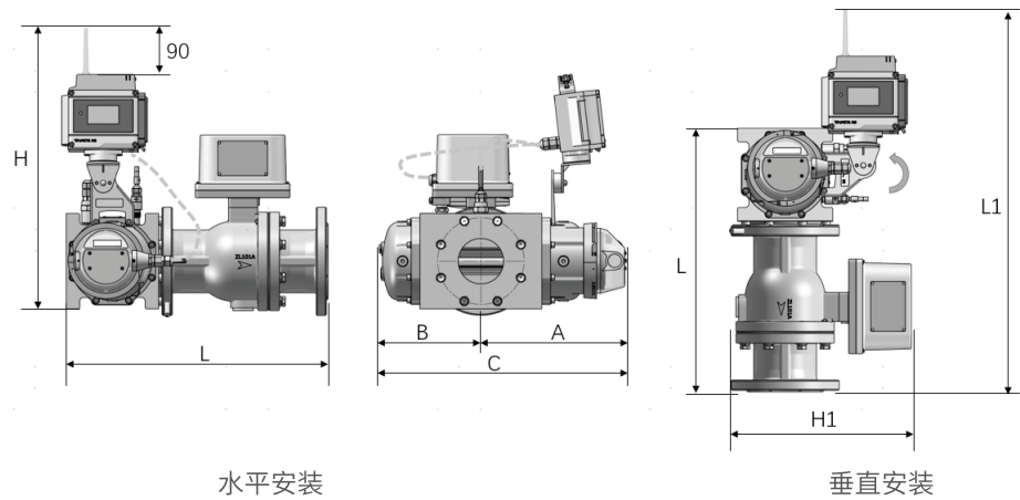
图 5-12 TEP-G □ -2-M
