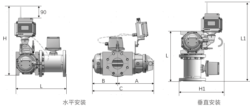
图 5-11 TEP-G □ -2
