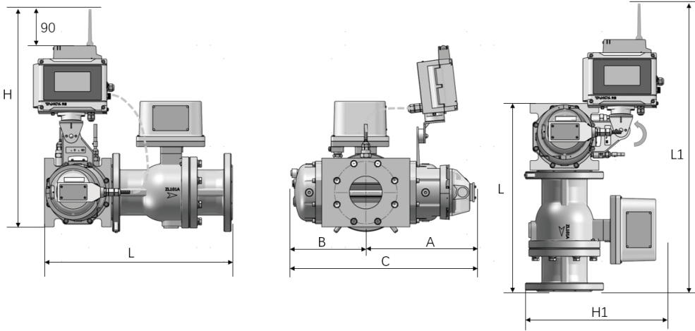
水平安装
