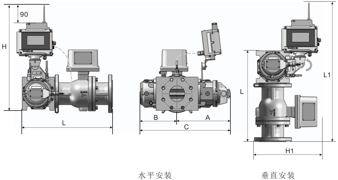
图5-9 G□/TFC-□/TCVL-M-□-R
