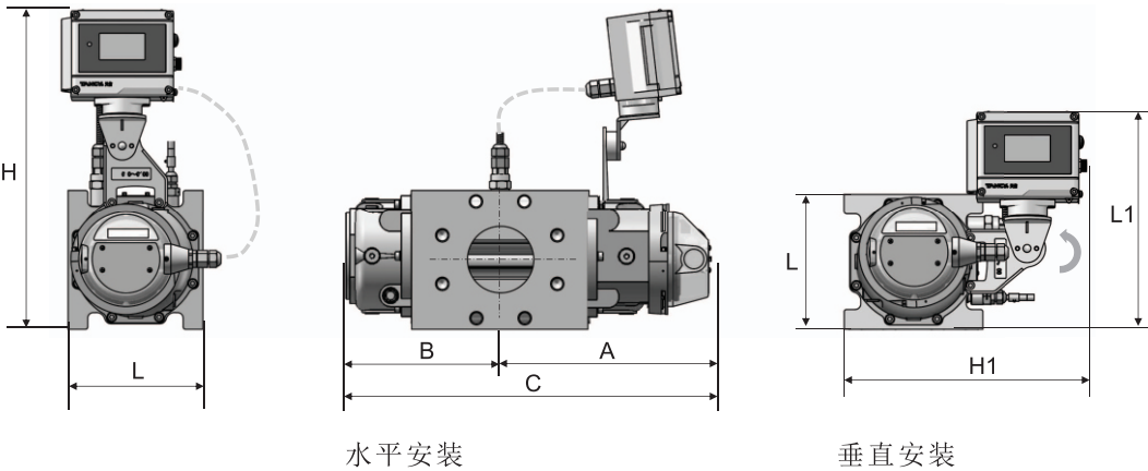
图5-4 G□/FCM-V
